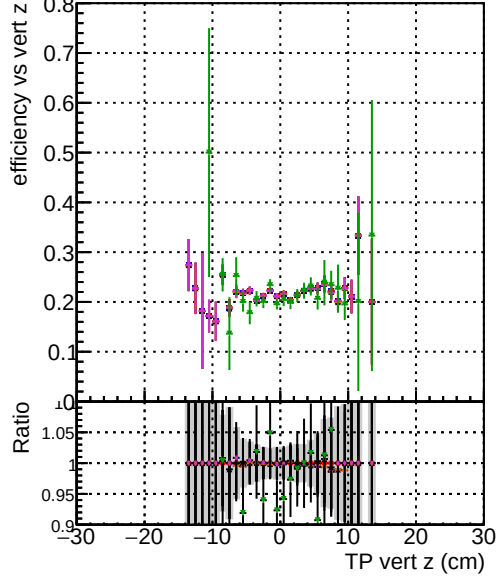
Efficiency vs vert z BGM original original vector 1000evt BGM fitted4 1000evt BGM fitted4 5000evt BGM fitted4 10000evt BGM fit cpeOK SORTRZZ 1000evt BGM fit cpeOK SORTRZZ TESTOUTLIER2 1000evt
