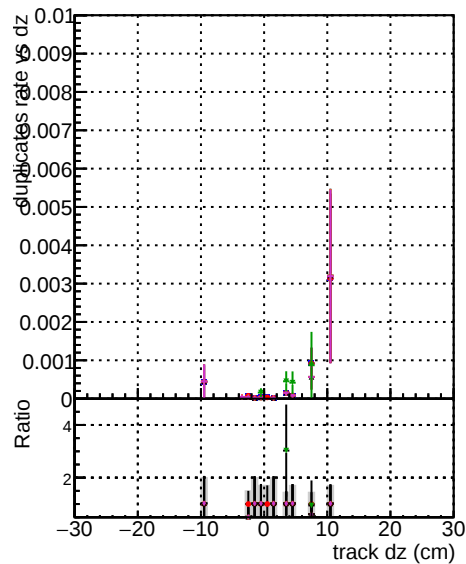
SPOUTLIER 1000evt
