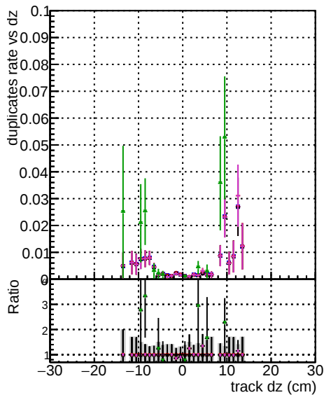
OUTLIER 1000evt
