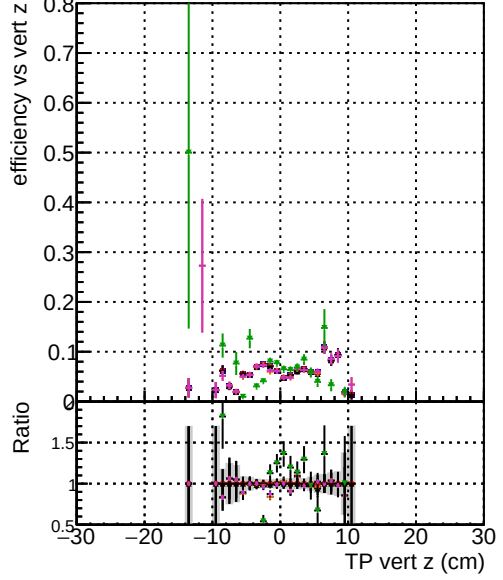
Efficiency vs vert z Legend: - BGM original original vector 1000evt - BGM fitted 4 1000evt - BGM fitted 2 1000evt - BGM fitted cpeok SORTRZZ 1000evt - BGM fitted cpeok SORTRZZ TESTOUTLIER 1000evt
