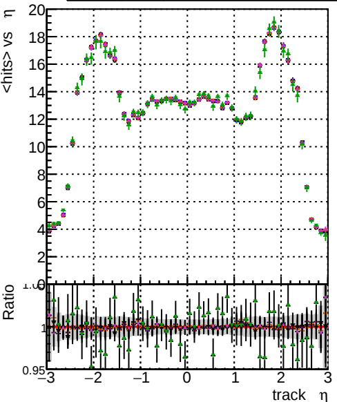
mean hits vs \eta Legend: BGM original original vector 1000evt, BGM fitted 1000evt, BGM fit cpeok SORTZZ 1000evt, BGM fit cpeok SORTZZ TESTOUTLIER 1000evt
