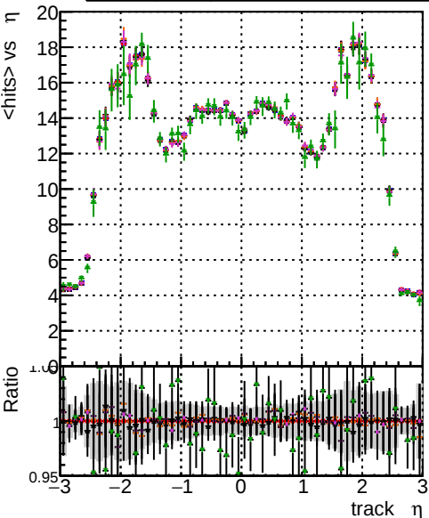
mean hit \eta BDW original original vector 1000evt BDW fitted 1000evt BDW fit cpeok SORTRZZ 1000evt BDW fit cpeok SORTRZZ TESTOUTLIER 1000evt
