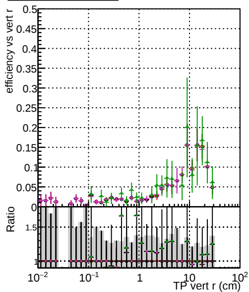
DOM-original-originalvector_1000evt
