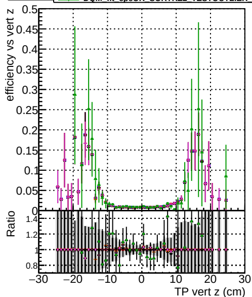
Efficiency Legend: DOM original original vector 1000evt DOM fitted 4 1000evt DOM fit cpeck 1000evt DOM fit cpeck SORTB22 1000evt DOM fit cpeck SORTB22 TESTOUTLIER 1000evt
