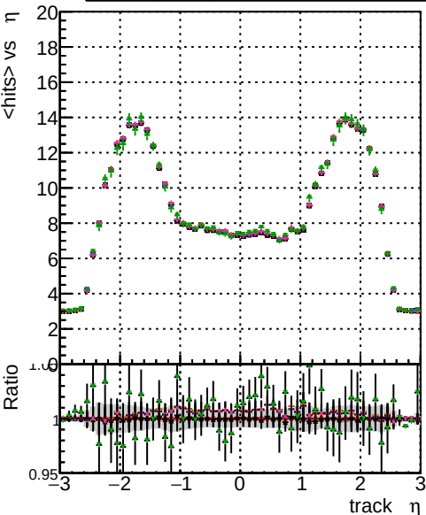
mean hits vs \eta Legend: BGM original original vector 1000evt, BGM fitted 4 1000evt, BGM fitted 22 1000evt, BGM fit cpeok SORTZZ 1000evt, BGM fit cpeok SORTZZ TESTOUTLIER 1000evt
