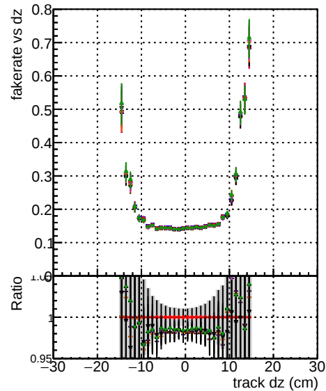
Fake rate vs dz Legend: DOM original_1000evt original_1000evt DOM IL CERN 5017Rz_1000evt
