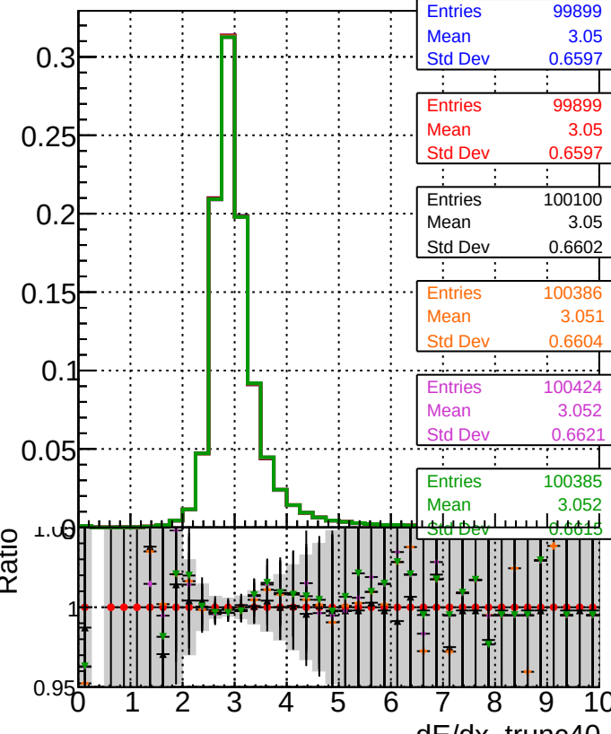
dE/dx estimator 2
