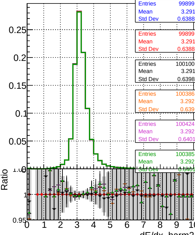
dE/dx estimator 1
