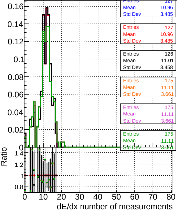
DOM original originalvector_1000evt DOM fitted4_1000evt DOM fit nocpe_1000evt DOM fit cpeOK_1000evt DOM fit cpeOK SORTRZ_1000evt
