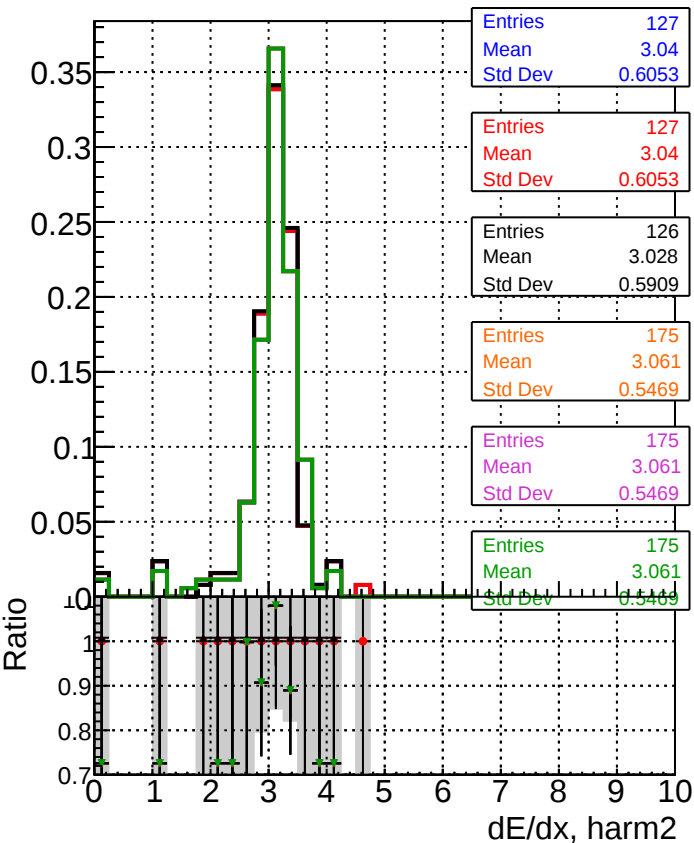
DOM original originalvector_1000evt DOM fitted4_1000evt DOM fit nocpe_1000evt DOM fit cpeOK_1000evt DOM fit cpeOK SORTRZ_1000evt
