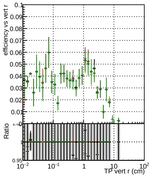
BGM original original vector 1000evt BGM fitted 4 1000evt BGM fit noedge 1000evt BGM fit cpeok SORTZ 1000evt
