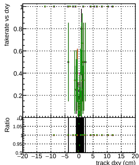
Fake rate vs d Legend: DOM original_1000evt DOM original_5000evt DOM original_10000evt DOM IL Check 5000evt DOM IL Check 10000evt
