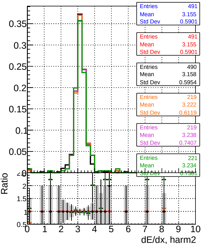
dE/dx estimator 1 DOM original originalvector_1000evt DOM fitted4_1000evt DOM fit nocpe_1000evt DOM fit cpeOK_1000evt DOM fit cpeOK SORTRZ_1000evt
