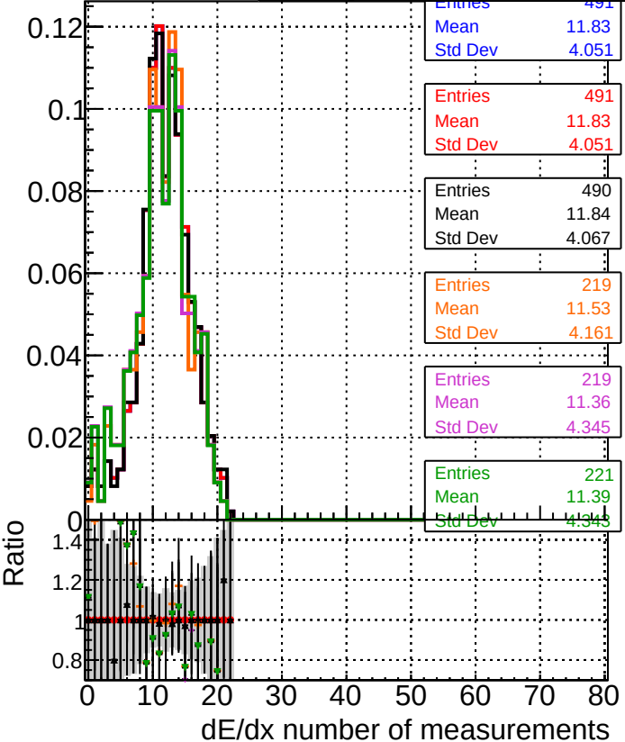
dE/dx estimator 1 DOM original originalvector_1000evt DOM fitted4_1000evt DOM fit nocpe_1000evt DOM fit cpeOK_1000evt DOM fit cpeOK SORTRZ_1000evt
