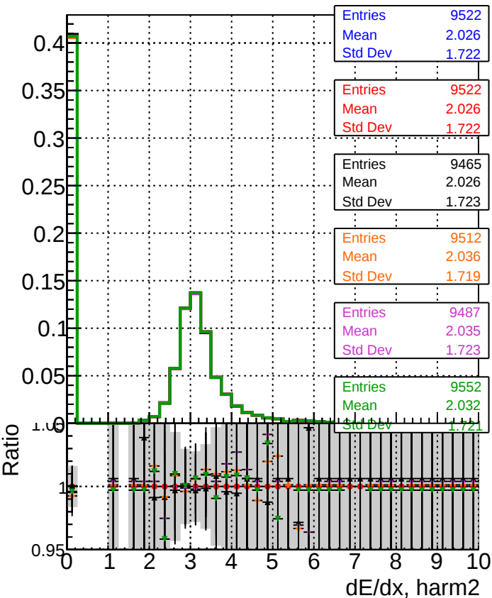
dE/dx estimator 3 Legend: DOM original originalvector_1000evt DOM original_1000evt DOM fitted4_1000evt DOM fit nocpe_1000evt DOM fit cpeOK_1000evt DOM fit cpeOK SORTRZ_1000evt
