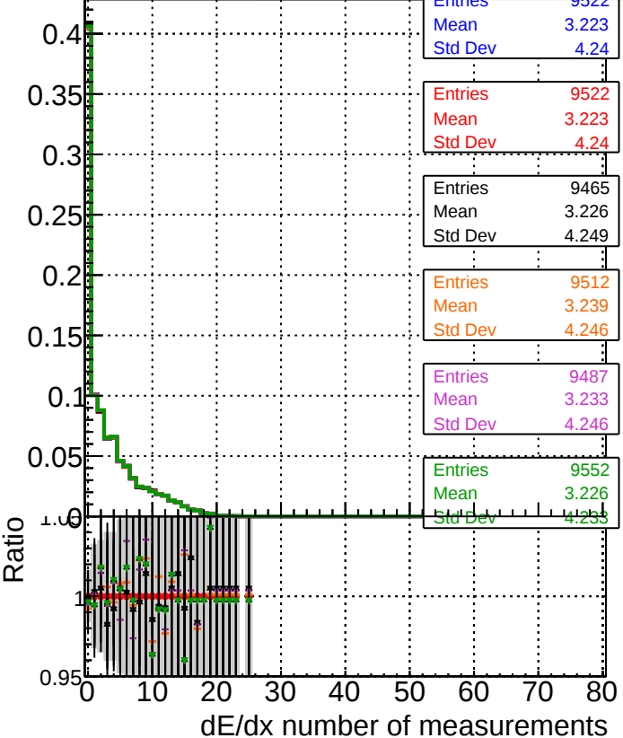
dE/dx estimator 3 Legend: DOM original originalvector_1000evt DOM original_1000evt DOM fitted4_1000evt DOM fit nocpe_1000evt DOM fit cpeOK_1000evt DOM fit cpeOK SORTRZ_1000evt
