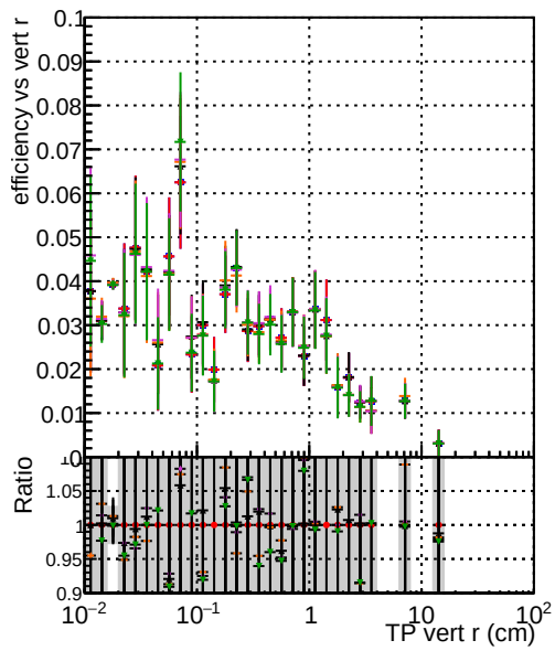
Legend for Efficiency vs vertpos and fake+duplicates vs vert r: — original data vector 1000evt — fitted 4 1000evt — fit nope 1000evt — fit cpeok SORTRZ 1000evt
