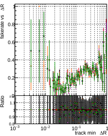
Fake rate vs \Delta R (track, jet) 1000evt 10000evt 1000evt 100evt 10evt 1evt
