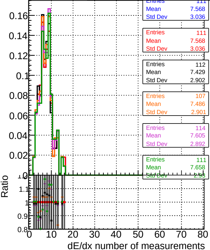
dE/dx estimator 1 Legend: DOM original originalvector_1000evt DOM original_1000evt DOM fitted4_1000evt DOM fit nocpe_1000evt DOM fit cpeOK_1000evt DOM fit cpeOK SORTRZ_1000evt
