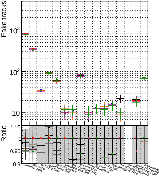
Number DQM fit noCPE 1000evt DQM fit cpeOK 1000evt DQM fit cpeOK SORTRZ 1000evt
