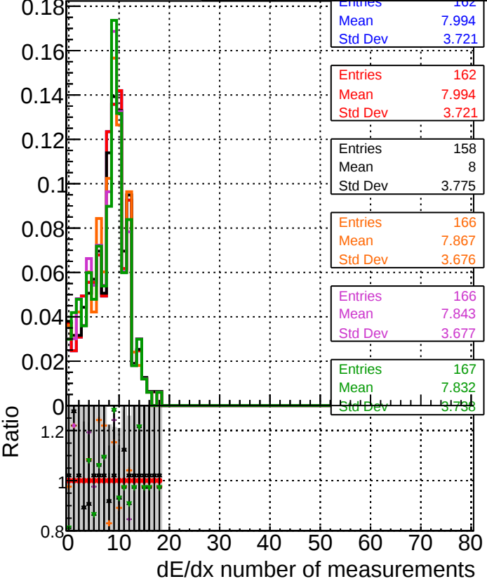
dE/dx estimator 1 DOM original originalvector_1000evt DOM original 1000evt DOM fitted4 1000evt DOM fit nocpe 1000evt DOM fit cpeOK 1000evt DOM fit cpeOK SORTRZ 1000evt
