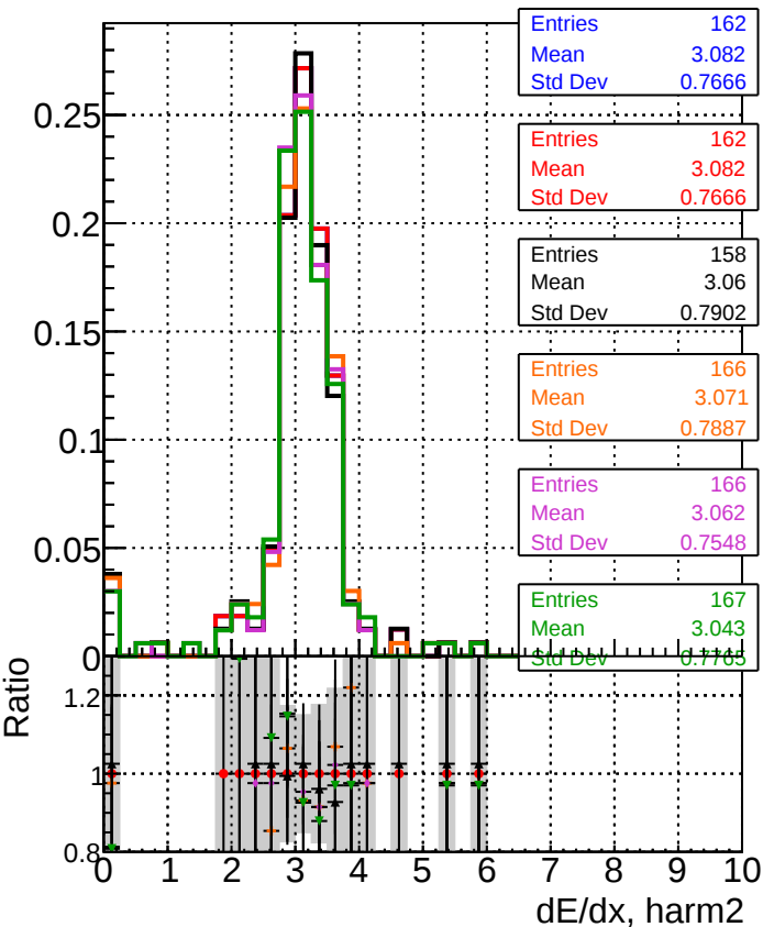
dE/dx estimator 1 DOM original originalvector_1000evt DOM original 1000evt DOM fitted4 1000evt DOM fit nocpe 1000evt DOM fit cpeOK 1000evt DOM fit cpeOK SORTRZ 1000evt
