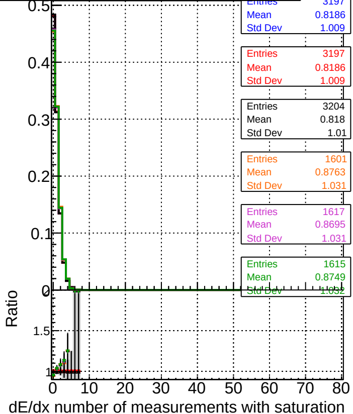
dE/dx estimator 2
