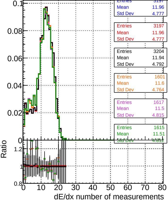
dE/dx estimator 1
