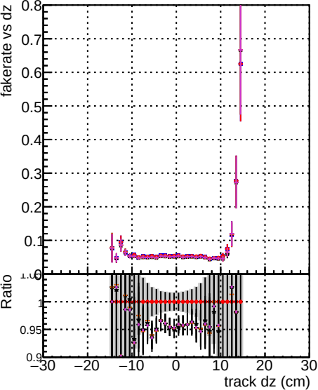
Fake rate vs dz DOM original original vector original 1000evt original 10000evt original 100000evt
