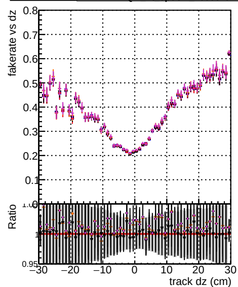
Fake rate vs dz DOM original 1000evt DOM original 1000evt DOM fit 1000evt
