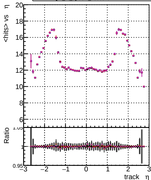
mean hits vs \eta DOM original 1000evt DOM original 1000evt DOM fit dca 1000evt DOM fit ncpk 1000evt DOM fit cpeOK 1000evt
