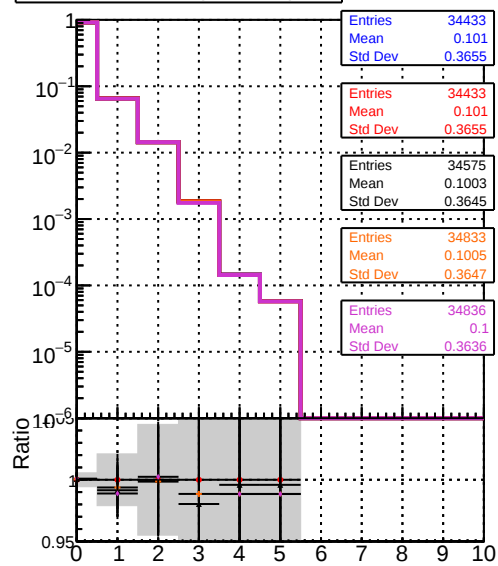
mean hits vs \eta DOM original originalvector_1000evt DOM original_1000evt DOM fitted_1000evt DOM fit nocpe_1000evt DOM fit cpeOK_1000evt
