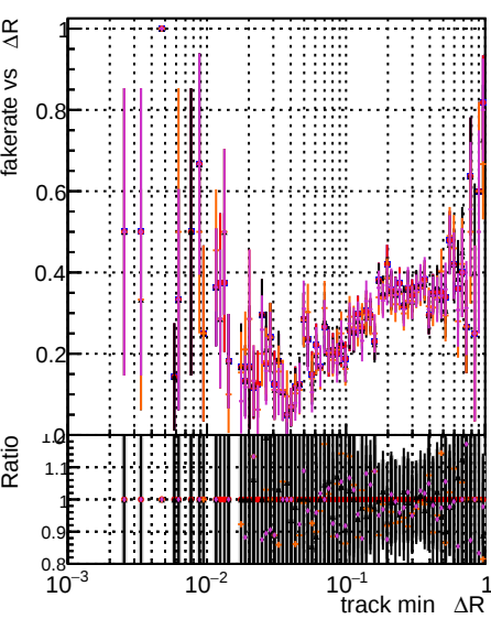
Fake rate vs \Delta R(\text{track, jet}) Legend: DOM original - original vector 1000evt DOM hit 1000evt DOM hit 1000evt DOM hit 1000evt DOM hit 1000evt
