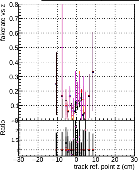
Fake rate vs vertpos DOM original original vector 1000evt DOM hit 1000evt DOM hit 1000evt DOM hit 1000evt DOM hit 1000evt
