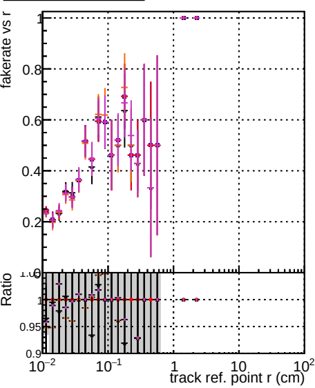
Fake rate vs v Legend: DOM original - 1000evt DOM hit - 1000evt DOM hit - 1000evt DOM hit - 1000evt DOM hit - 1000evt
