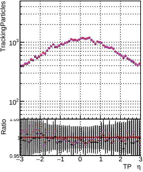
— DOM original originalvector_1000evt — DOM original_1000evt — DOM fit d4_1000evt — DOM fit nocpe_1000evt — DOM fit cpeOK_1000evt
