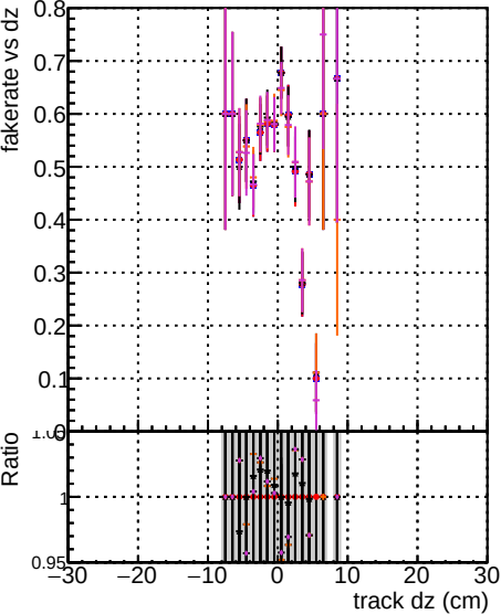
Fake rate vs dz DOM original-originalvector-1000evt DOM original-originalvector-10000evt DOM original-originalvector-100000evt DOM fit CDFK-10000evt
