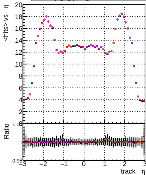
mean hits vs \eta DOM original 1000evt DOM original nocpe 1000evt DOM fit nocpe 1000evt DOM fit cpeOK 1000evt
