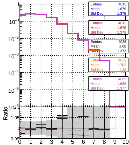
DOM original originalvector_1000evt DOM original_1000evt DOM fitadd_1000evt DOM fit nocpe_1000evt DOM fit cpeOK_1000evt
