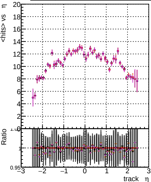
mean hits vs \eta DOM original 1000evt DOM original 1000evt DOM fitted 1000evt DOM fit nocpe 1000evt DOM fit cpeOK 1000evt
