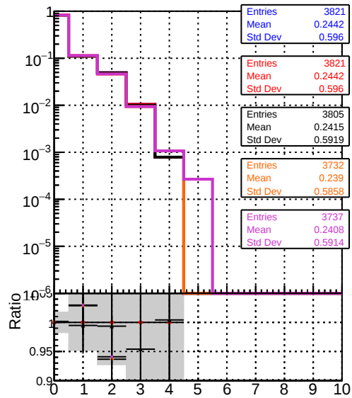
mean hits vs \eta DOM original 1000evt DOM original 1000evt DOM fit d4 1000evt DOM fit nocpe 1000evt DOM fit cpeOK 1000evt
