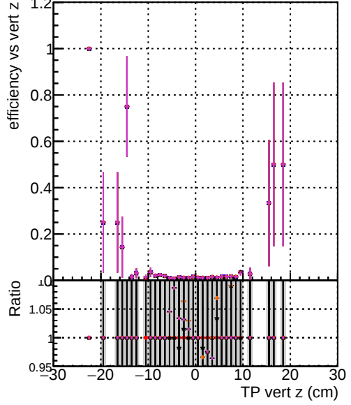
Efficiency vs vert z — DOM original originalvector_1000evt — DOM original_1000evt — DOM fitted4_1000evt — DOM fit nocpe_1000evt — DOM fit cpeOK_1000evt
