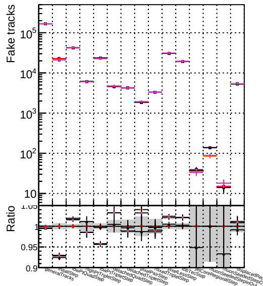
— DOM original 1000evt — DOM original 1000evt — DOM fit nocpe 1000evt — DOM fit cpeOK 1000evt
