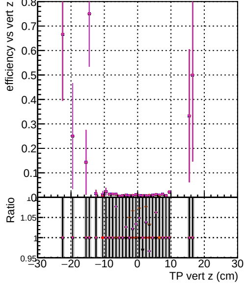
Efficiency vs vert z —•— DOM original originalvector_1000evt —•— DOM original_1000evt —•— DOM fitd4_1000evt —•— DOM fit nocpe_1000evt —•— DOM fit cpeOK_1000evt
