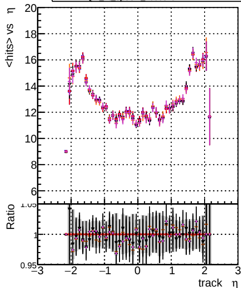
mean hits vs \eta DOM original 1000evt DOM original 1000evt DOM fitdd 1000evt DOM fit nocpe 1000evt DOM fit cpeOK 1000evt
