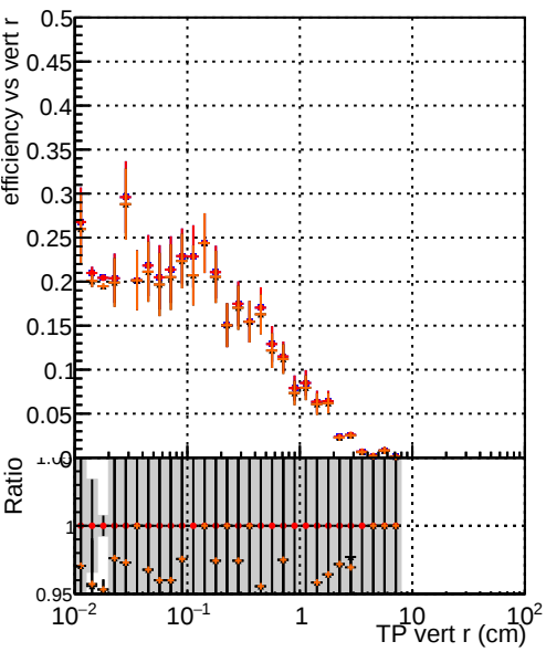
Efficiency vs TP vert r (cm) Legend: DOM original originalvector_1000evt DOM original_1000evt DOM fitted4_1000evt DOM fit_nocpe_1000evt
