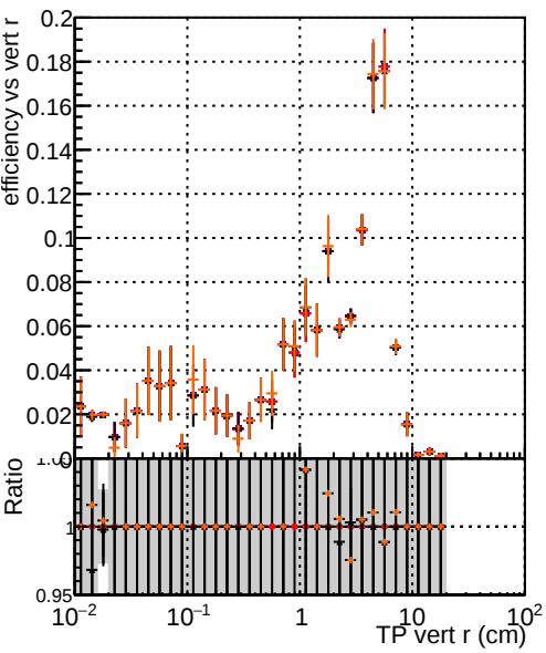
Efficiency vs vertpos DOM original originalvector_1000evt DOM original_1000evt DOM fitted4_1000evt DOM fit nocpe_1000evt
