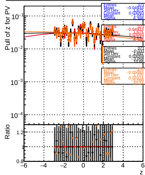
RecoPVAssoc2GenPVMatched_PulIZ
