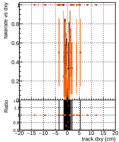
Fake rate vs d BSM original BSM original vector_1000evt BSM fit_1000evt BSM fit nocpe_1000evt
