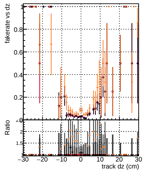
Fake rate vs d BSM original BSM original vector_1000evt BSM fit_1000evt BSM fit nocpe_1000evt
