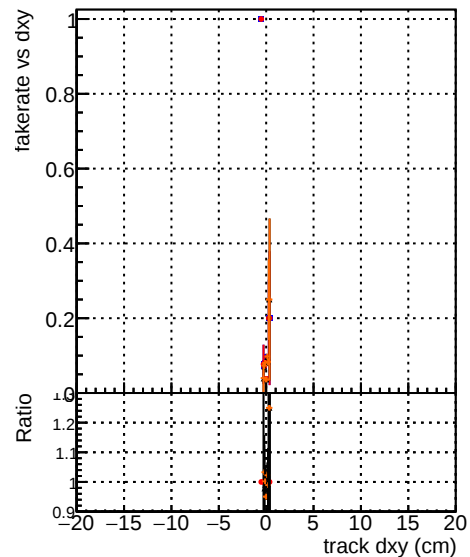
Fake rate vs d DOM original 1000evt DOM original vector 1000evt DOM fitted 1000evt DOM fit no cpe 1000evt
