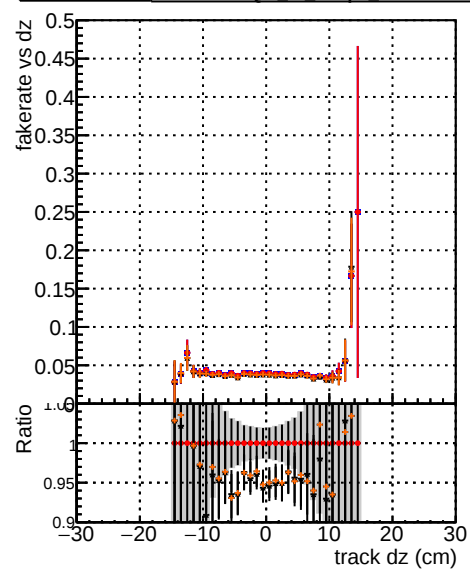
Fake rate vs d DOM original 1000evt DOM original vector 1000evt DOM fitted 1000evt DOM fit no cpe 1000evt
