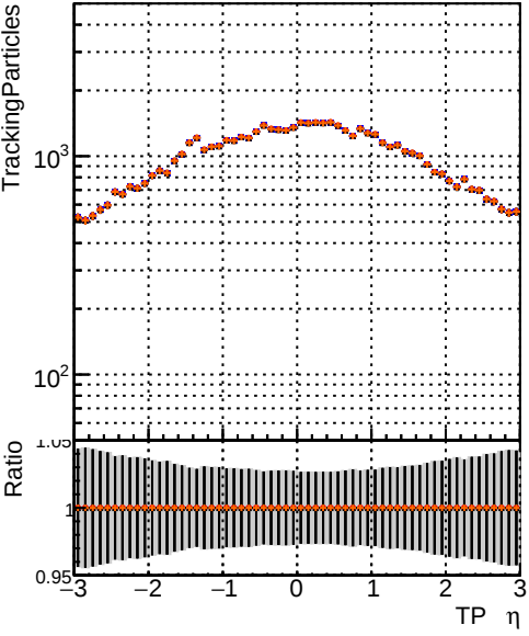
DQM original originalvector_1000evt DQM original_1000evt DQM fitted4_1000evt DQM fit_nocpe_1000evt
