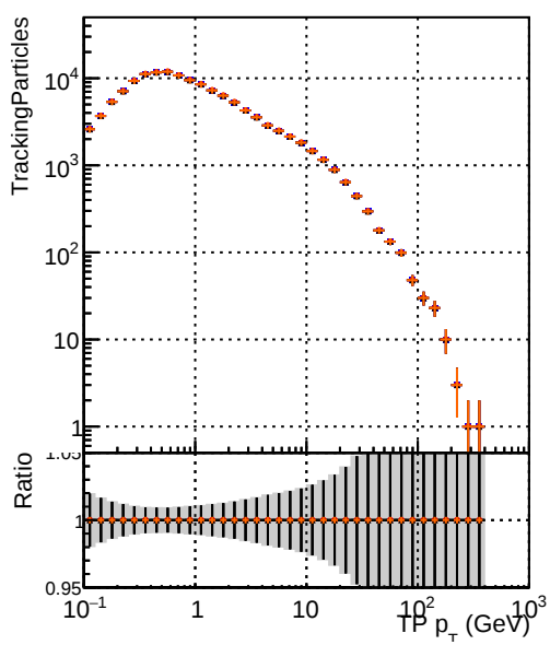
DQM original originalvector_1000evt DQM original_1000evt DQM fitted4_1000evt DQM fit_nocpe_1000evt
