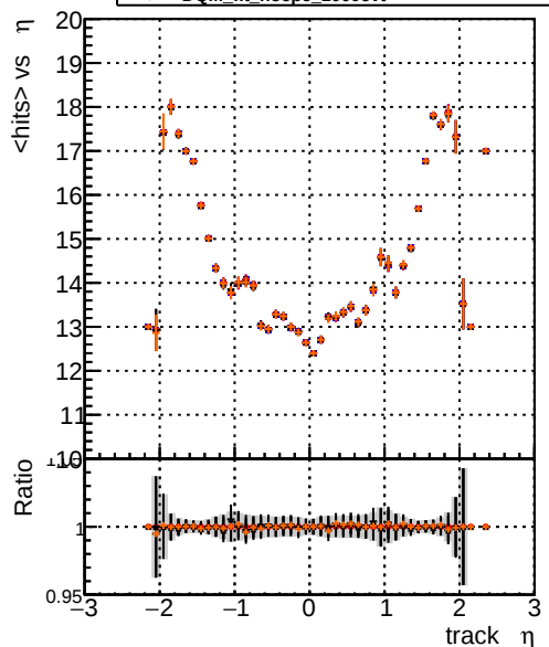
mean hits vs \eta DOM_original_1000evt DOM_original_1000evt DOM_fitted4_1000evt DOM_fit_nocpe_1000evt
