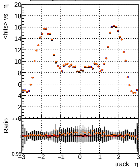
mean hits vs \eta DOM_original_originalvector_1000evt DOM_original_1000evt DOM_fitted4_1000evt DOM_fit_nocpe_1000evt
