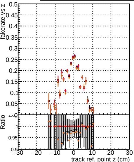
Fake rate vs vertpos DOM original original vector 1000evt DOM fitted 1000evt DOM fit nocpe 1000evt
