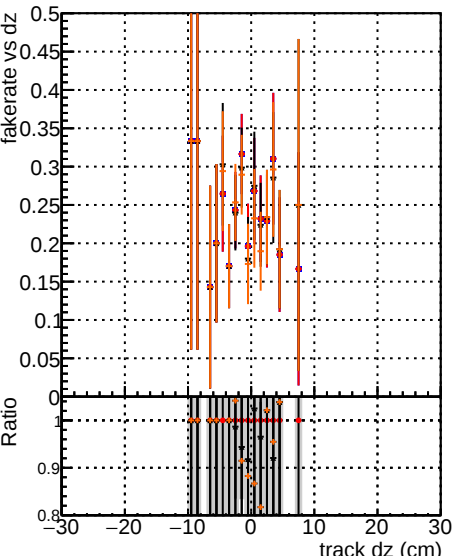
Fake rate vs dz Legend: DSM original - originalvector 1000evt DSM original - originalvector 10000evt DSM original - originalvector 100000evt DSM fit - fit 1000evt DSM fit - fit 10000evt DSM fit - fit 100000evt
