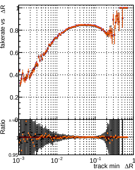
Fake rate vs \Delta R (track, jet) Ratio DQM original original vector 1000evt DQM fitted 1000evt DQM fit nocpe 1000evt
